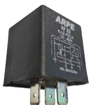
RELÉ PISCA 4 TERMINAIS S/ SUPORTE (Rp52) - ARPE
