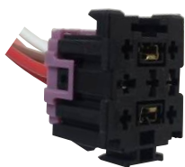
SOQUETE P/ RELÉ 5 TERMINAIS C/ CHICOTE (SOQ1512/24) - ARPE
