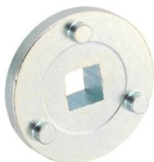
Arruela de 39mm para recuar o êmbolo da pinça de freio VW Passat 2005 em diante (usar com a ferramenta nº 12 104)
