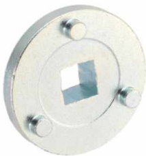
Arruela de 39mm para recuar o êmbulo da pinça de freio VW Passat 2005 em diante (usar com a ferramenta n° 12 104)
