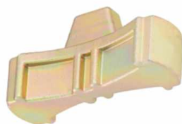
Ferramenta para sincronizar as polias das árvores de comando de válvulas do motor AT 1.0 16V (aspirado ou turbo) do Gol, Parati e Polo Classic
